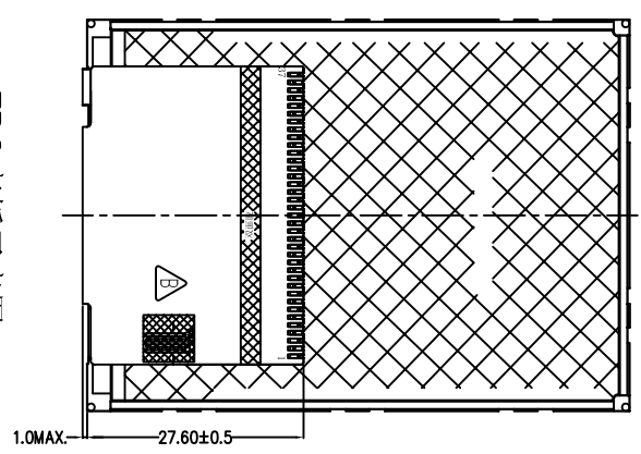
FPC弯折示意图 (展开出货)
